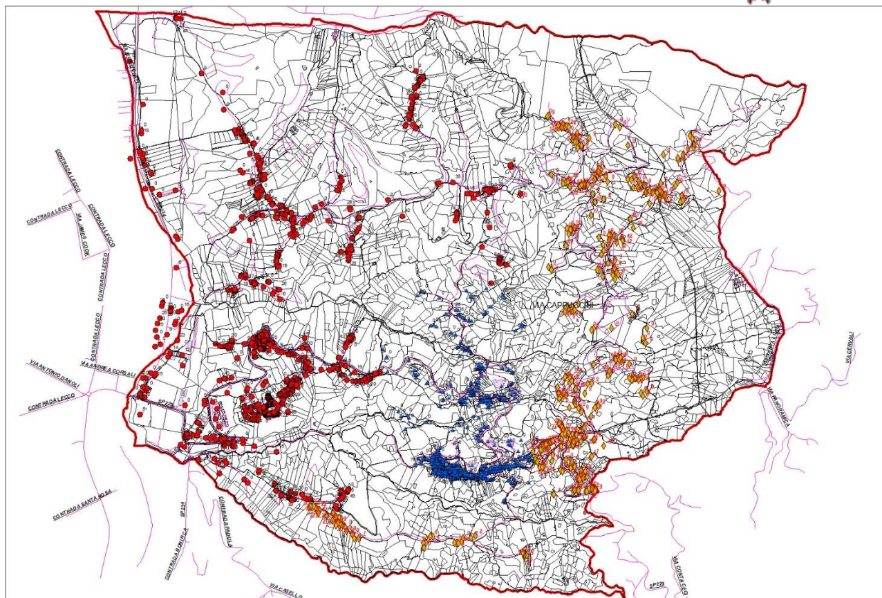
Fig. 3 – Castiglione Cosentino - Planimetria con relativo database interrogabile a video degli accessi con numerazione civica assegnata. (ogni colore è riferito ad un differente rilevatore)
